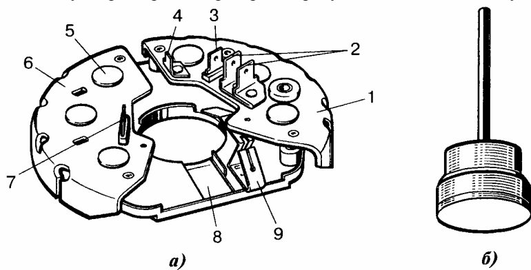
Рис. 16. Выпрямительный блок генераторов K I, NI фирмы Bosch а - выпрямительный блок, б - диод выпрямительного блока: 1 - положительный теплоотвод; 2,8 - выводы "В+" генератора; 3 - вывод "D+" генератора; 4 - вывод "+" для конденсатора; 5 - запрессованный диод; 6 - отрицательный теплоотвод; 7 - вывод "W" генератора; 9 - пружинный вывод "D+"
