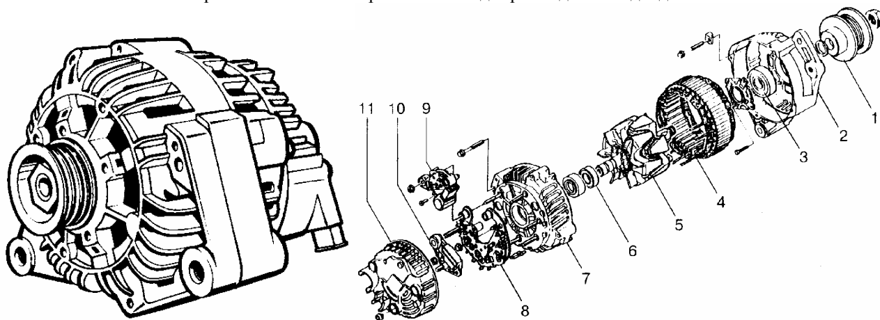
Рис.22. Внешний вид компактных генераторов A13VT концерна Valeo
